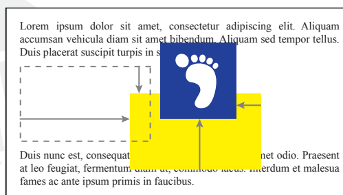
Figura 3.7: Elemento com position diferente de static utilizado como referência
