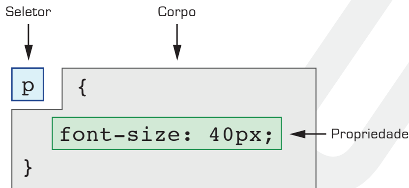
Figura 3.3: Estrutura de uma regra CSS
